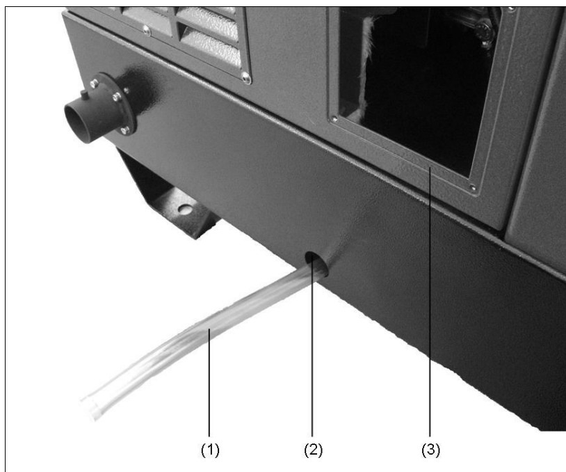
Abb. 7-1: Öl ablassen
