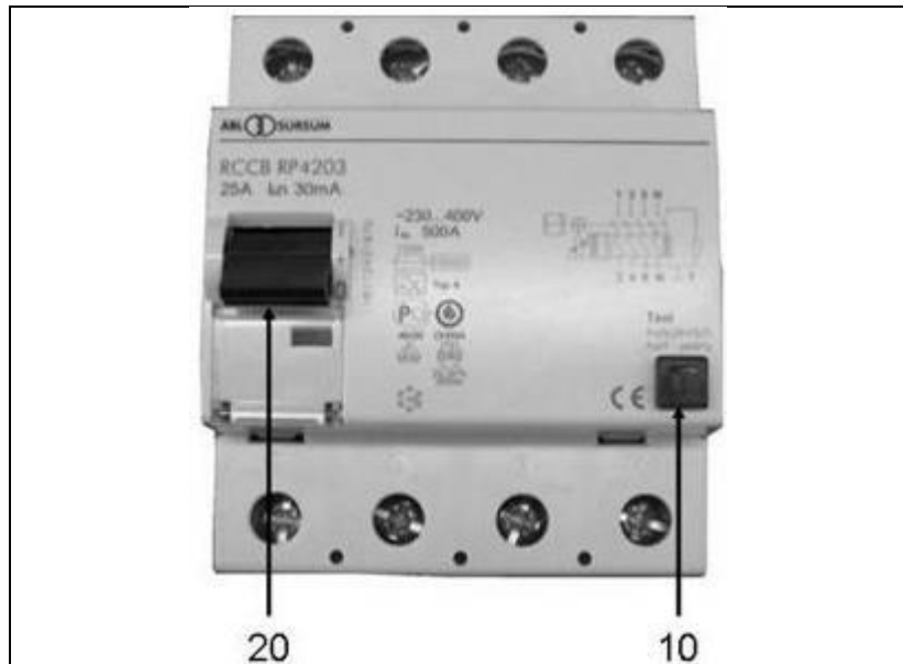
Abb. 5-2: FI- Schutzschalter
