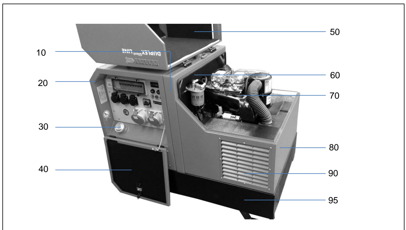
Abb. 10-1: Ersatzteile der Abgas bzw. Generatorseite
