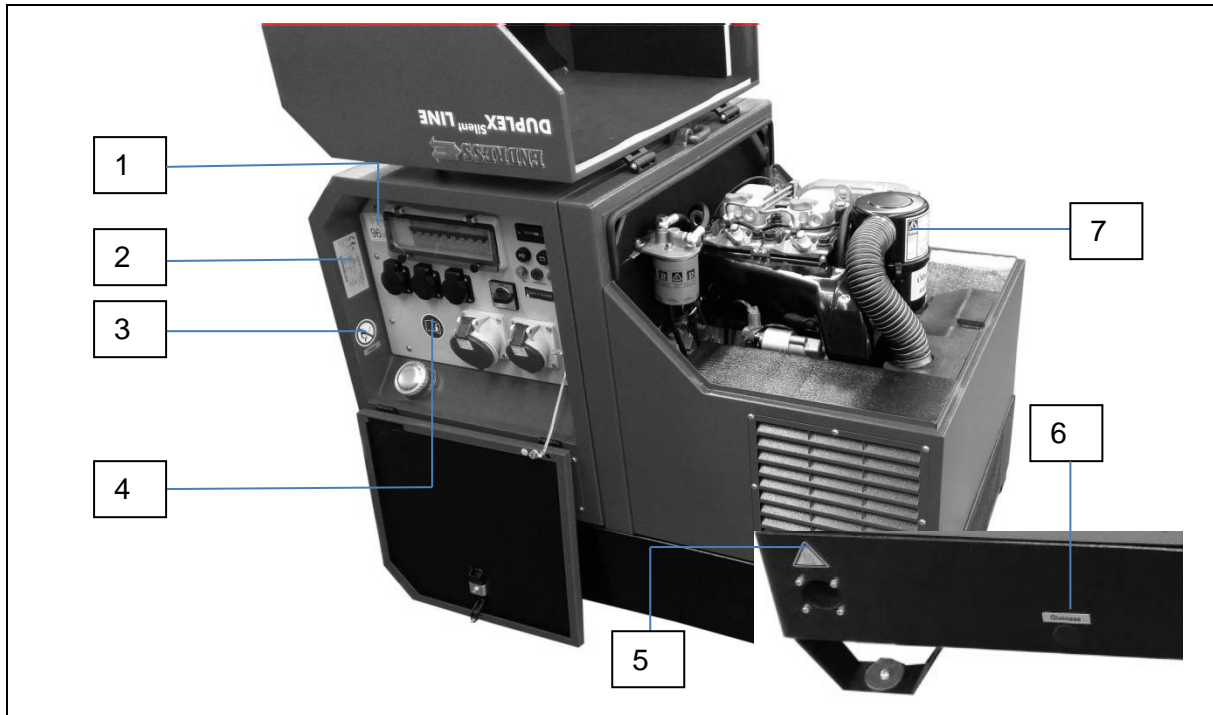
Abb. 2-1: Kennzeichnungen am Stromerzeuger
